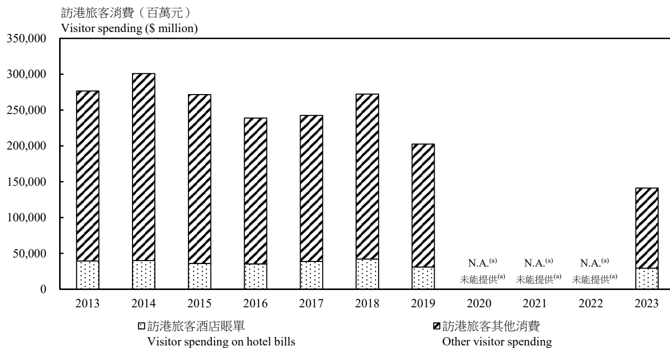
圖 14.2(a) 訪港旅客消費 (a)(b) Chart 14.2(a) Visitor spending (a)(b)
